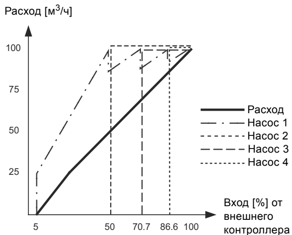
Рис. 28 Регулировочная характеристика для MPC-F в разомкнутом контуре
