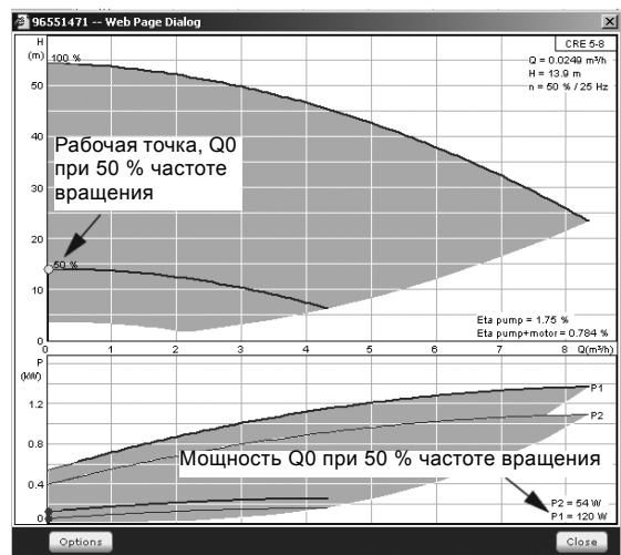
Рис. 91 Показание мощности Q0 при 50 % частоте вращения (WebCAPS)
