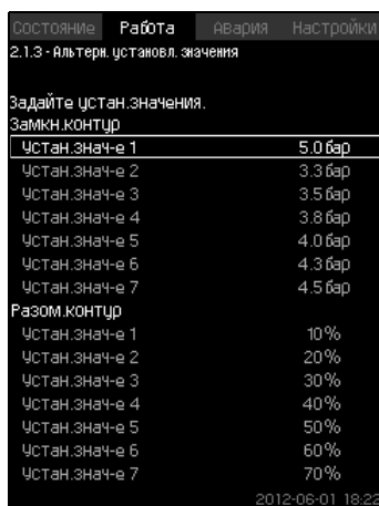
Рис. 30 Альтерн. установл. значения
