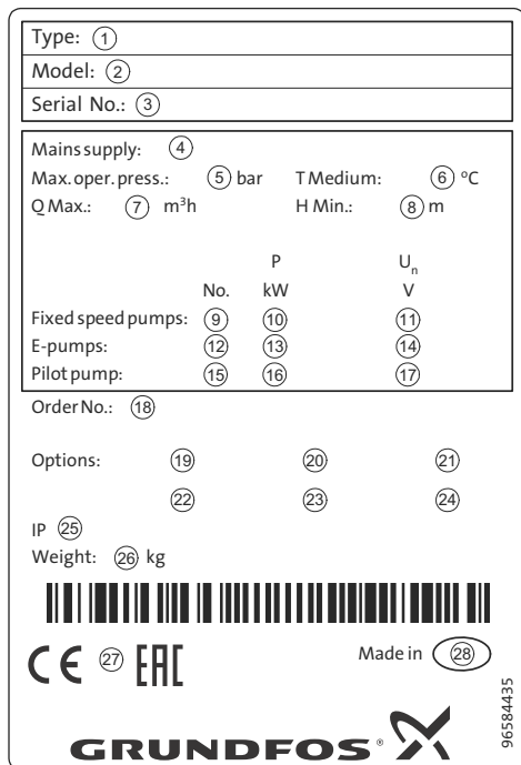
Рис. 2 Фирменная табличка
