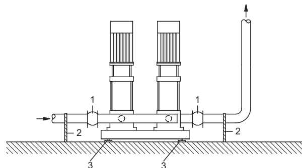
Рис. 5 Положение вибровставок, опор для труб и вибрационных опор
