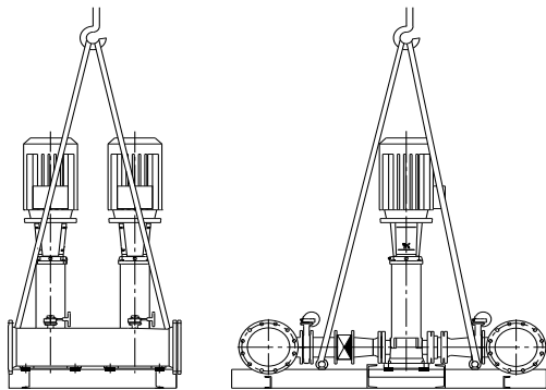
Рис. 4 Правильный подъем Hydro MPC XL
