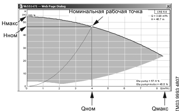
Рис. 89 Показание Qном, Hном, Hмакс и Qмакс (WebCAPS)
