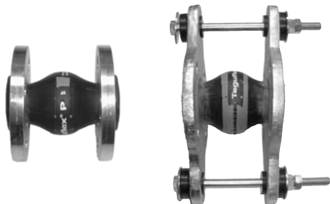
Рис. 6 Вибровставки с резиновыми прокладками без ограничительных стяжек и с ними
